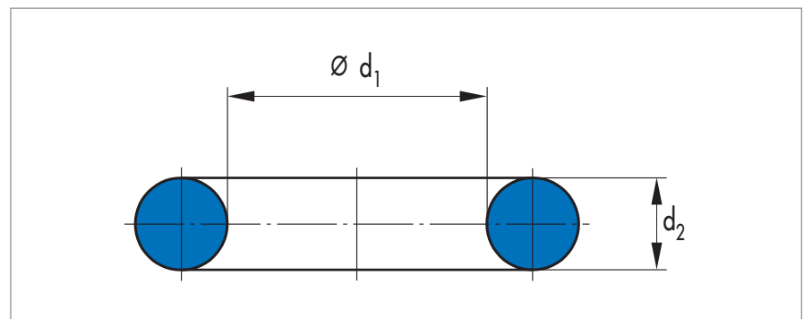
Abb. 2 Maßskizze
